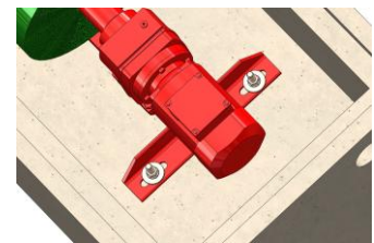
Abb. 22 Befestigung Rückrollvorrichtung
