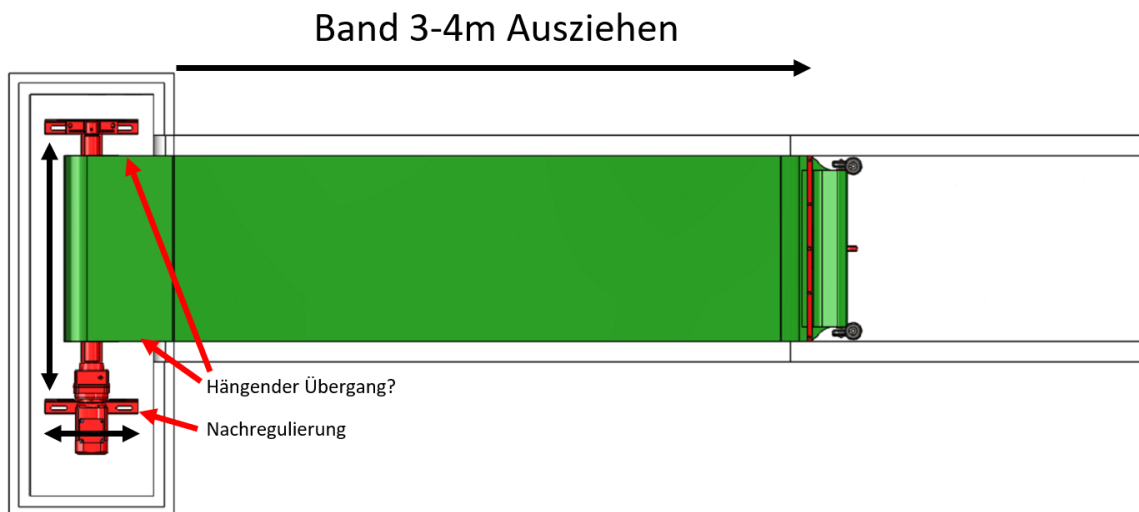
Abb. 24 Montage Rückrollvorrichtung
