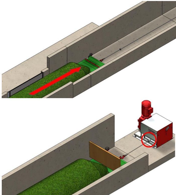
Abb. 36 Feedstar befüllen
