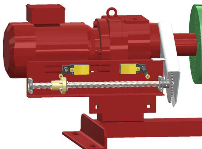
Abb. 9 Endabschaltung Rückrollvorrichtung
