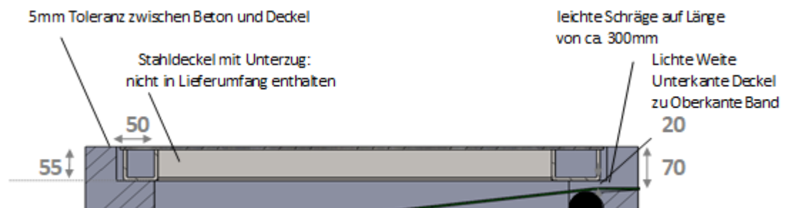
Abb. 6 Stahldeckel mit Unterzug (optional)
