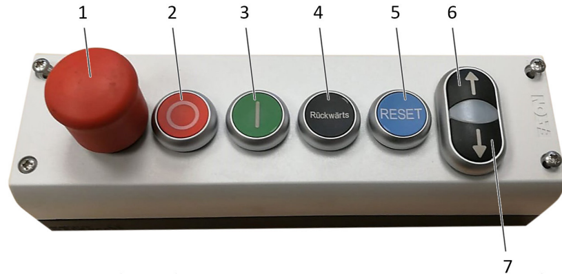
Abb. 5 Mobile Bedieneinheit
