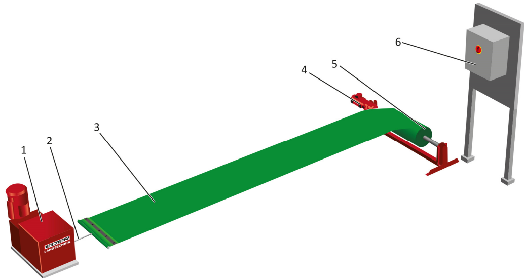
Abb. 2 Futterband, schematische Gesamtansicht
